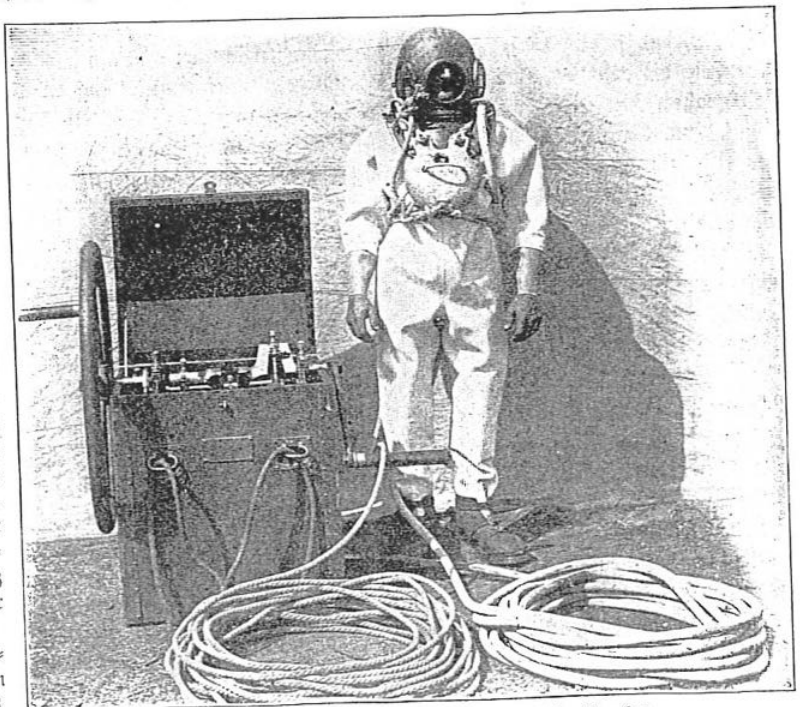
Mit Sicherheitsleine und Luftschlauch ausgerüsteter Taucher.
