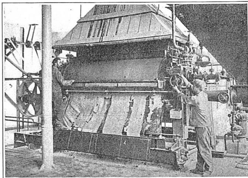
Eine Maschine, Kartoffelflocken und Kartoffelmehl zu bereiten.
