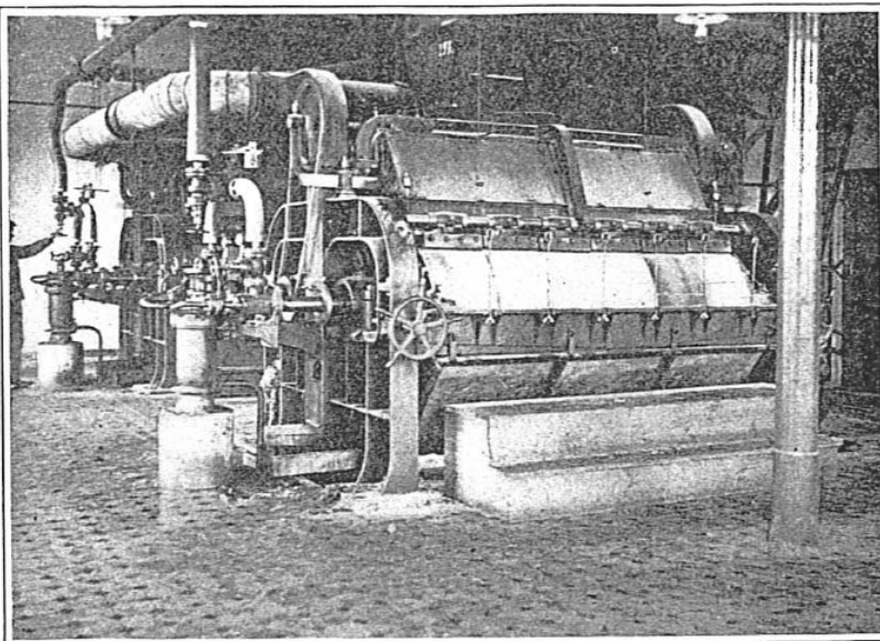
Eine Maschine zur Bereitung von Kartoffelschnitzeln.
