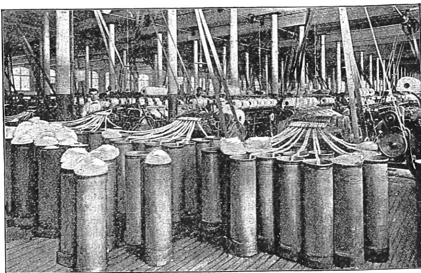
Die Vorspinnmaschine, welche die großen Stränge feiner spinnt.
