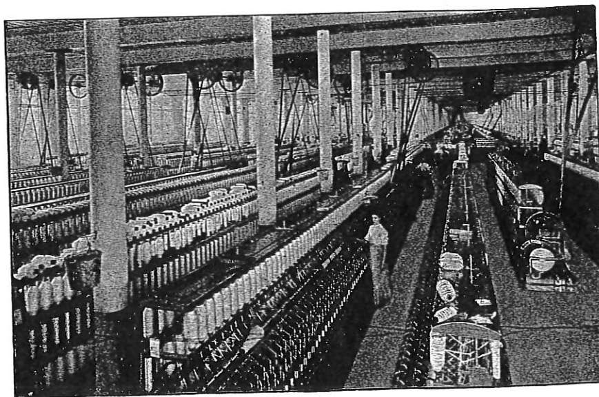
Spinnmaschinen für größere Spulen.
