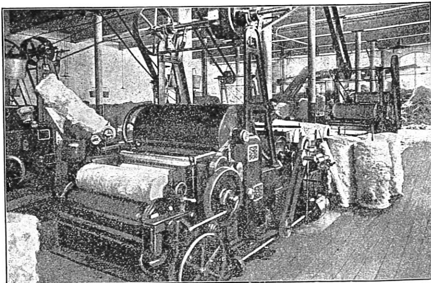
Die Wickelmaschine, welche die Baumwolle in Streifen aufrollt.
